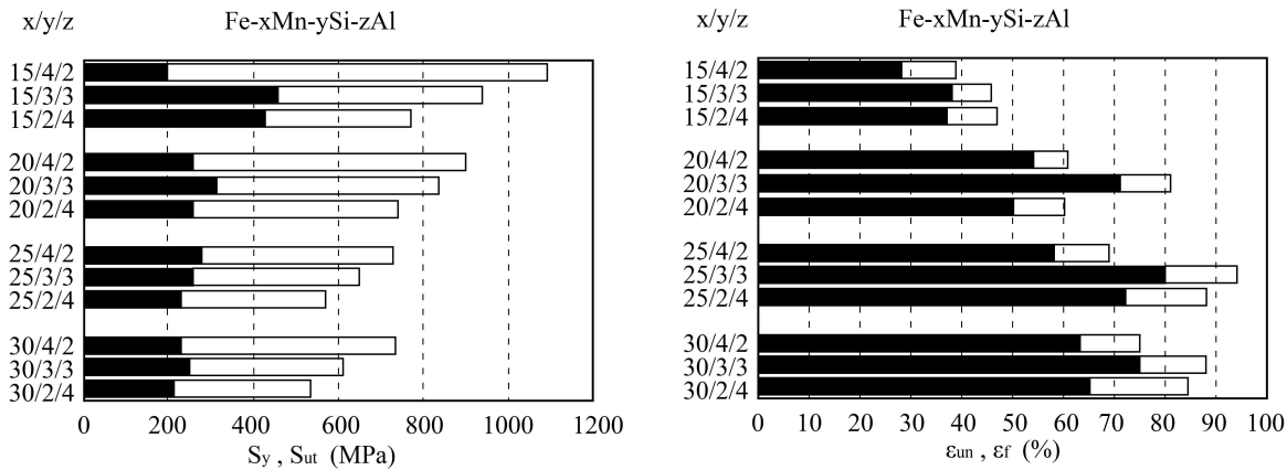
Figura 4. Resistencia y deformación relativa en función de la composición
