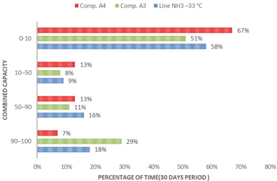
Figura 10. Análisis de capacidad para el circuito de -33 ° C.
