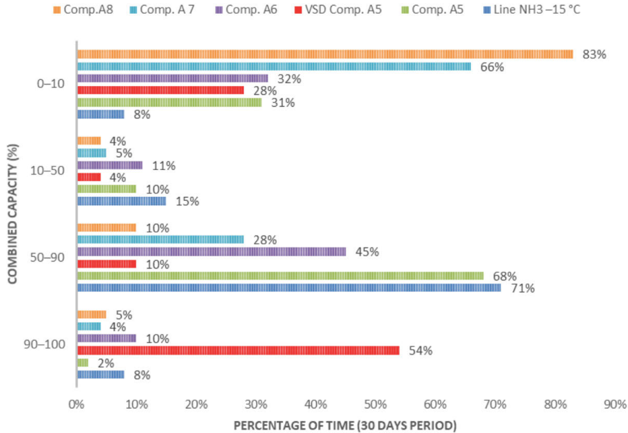
Figura 11. Análisis de capacidad para el circuito de -15 °C.
