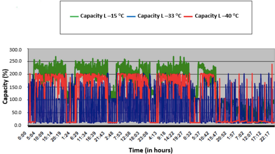
Figura 6. Perfil de funcionamiento de los diferentes grupos de compresores en el período estival.
