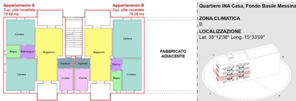
Figure 2. Le specifiche dell'unità immobiliare del blocco B5 del Quartiere INA Casa oggetto di attestazione di prestazione energetica. Source: Elaborazione delle autrici.
