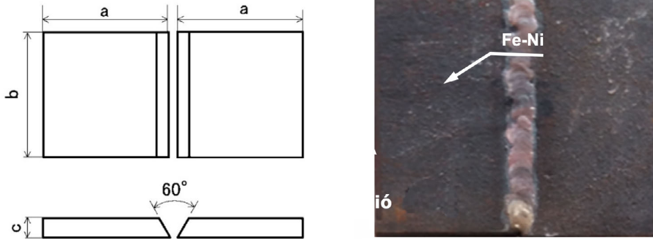
Figura 7. a) Preparación de probeta previo al soldado. b) Cupón soldado.
