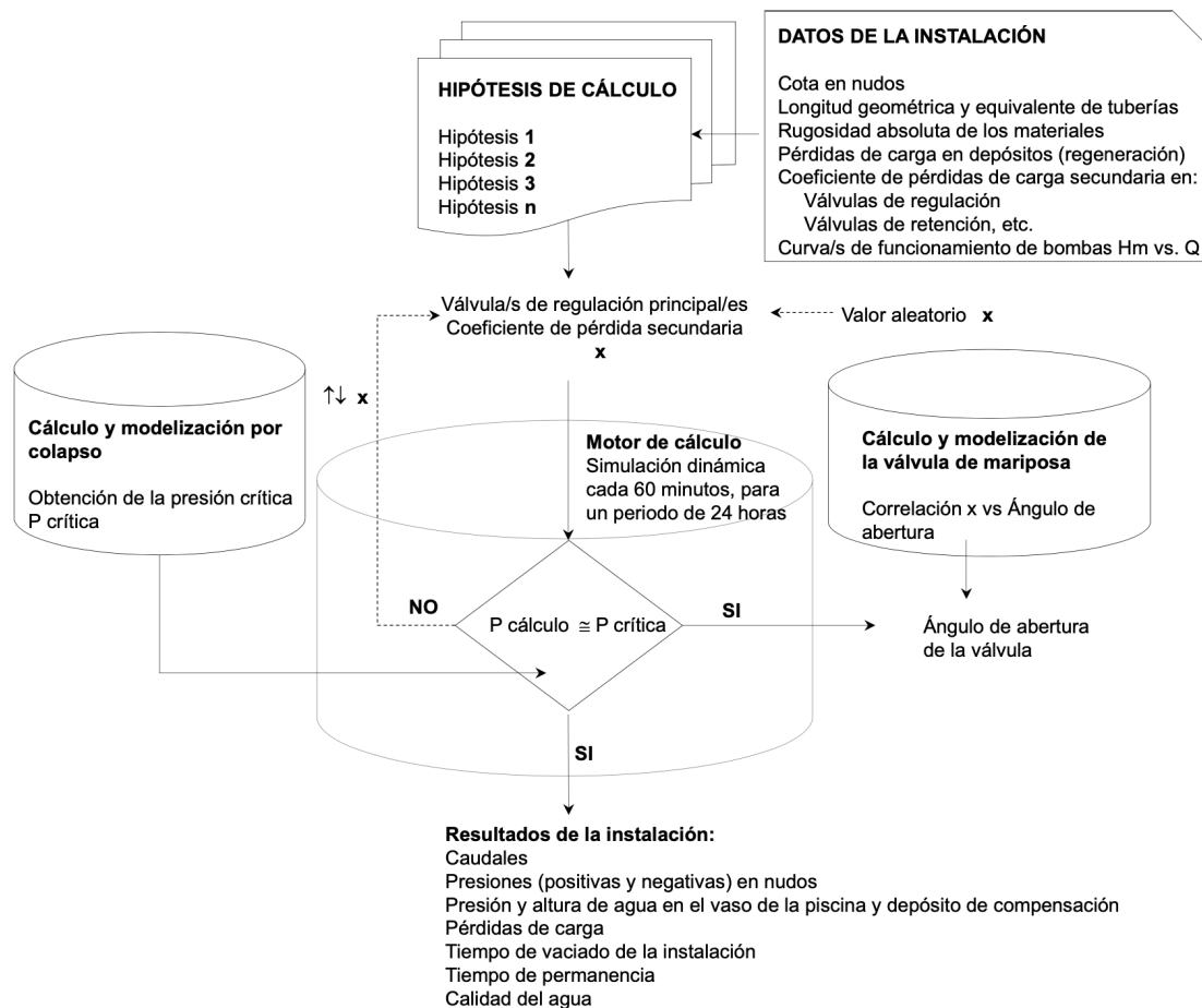
Figure 14. Algoritmo cálculo hidráulico
