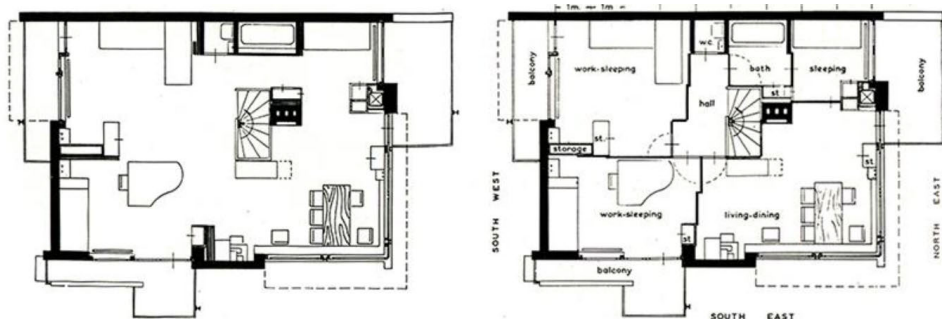
Figura 3. Gerrit Rietveld, Casa Schröder-Schröder, Utrecht, 1924, con la disposición abierta y cerrada de la planta superior con el concepto de flexibilidad arriba comentado.
