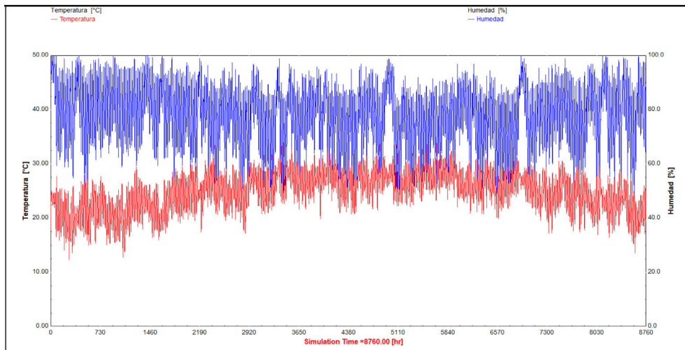
Figure 2. Evolución anual de la temperatura y humedad en Veracruz, México.
