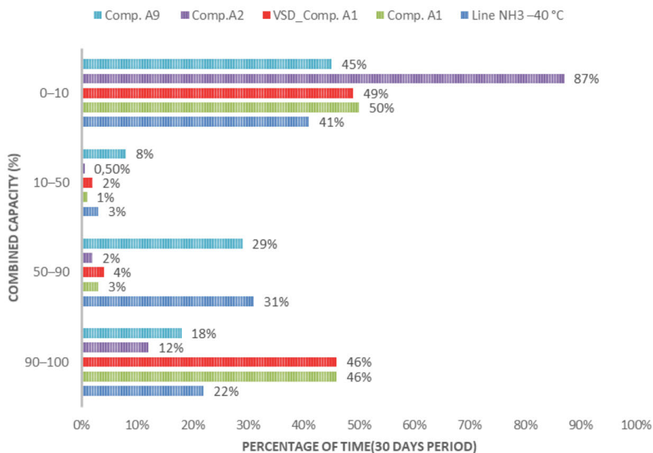
Figura 9. Análisis de capacidad para el circuito de -40 ° C.
